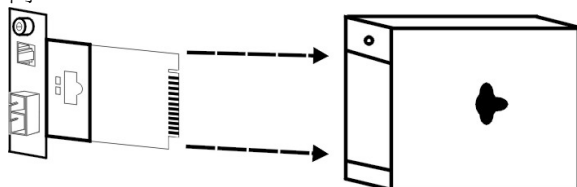
鬆開螺絲 取出媒介轉換電路板
